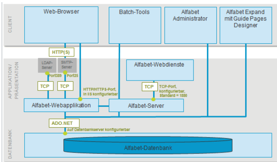
Abbildung: Von der Alfabet -Plattform verwendete Kommunikations-Ports
