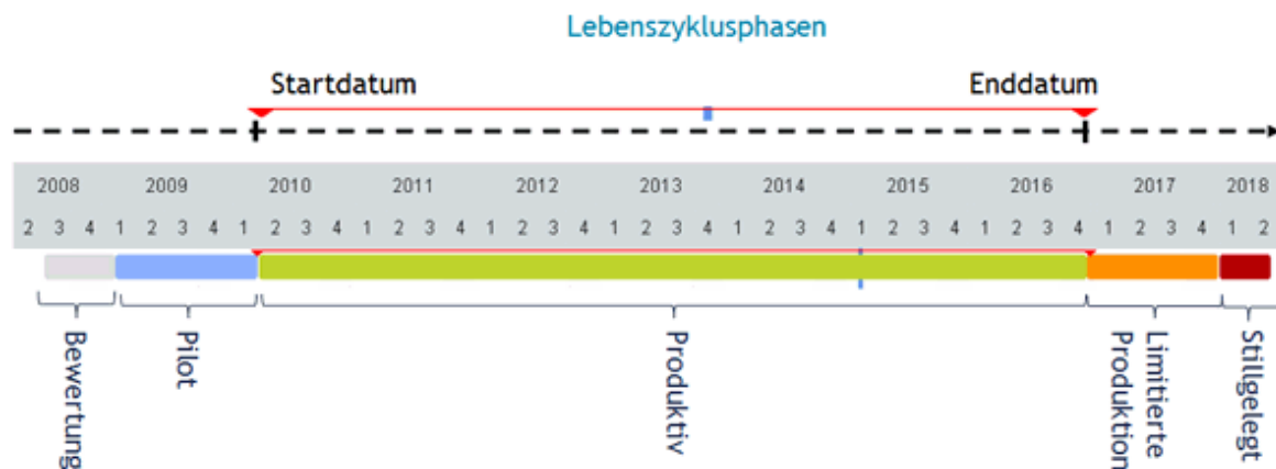
Abbildung: Applikationslebenszyklus
