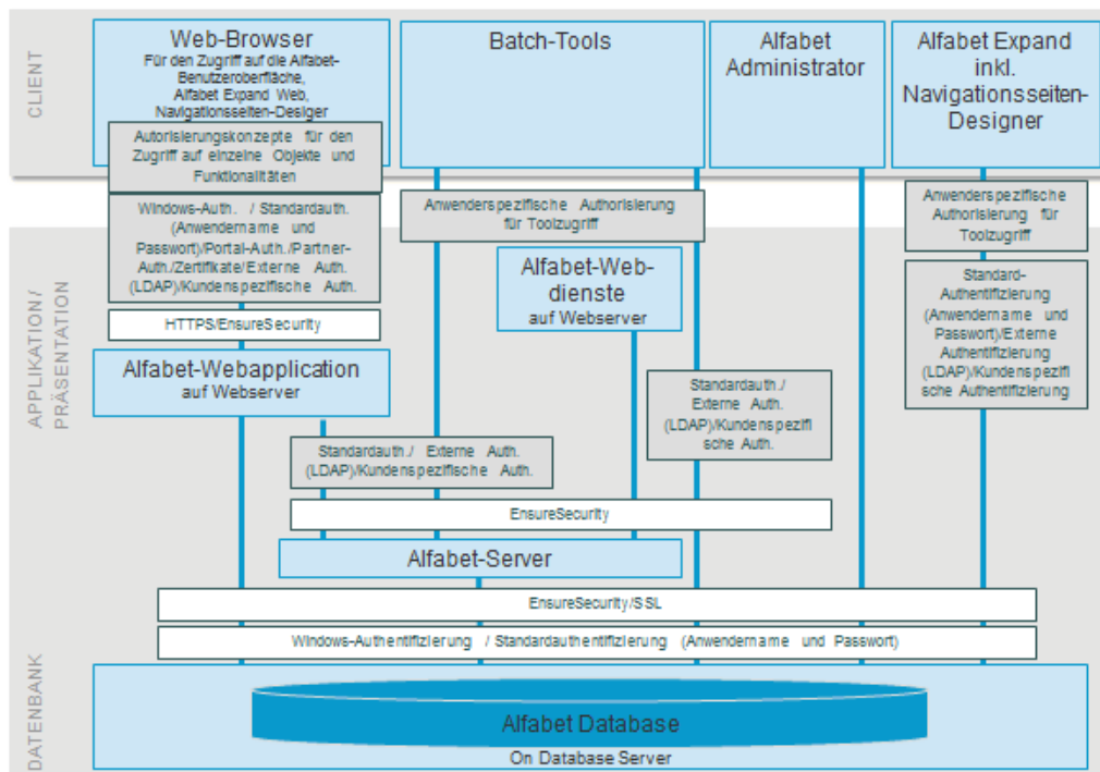
Abbildung: Sicherheitsmechanismen für den Zugriff auf Alfabet
