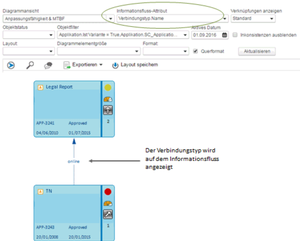
Abbildung: Anzeigen eines Informationsflussattributs über den Filter "Informationsfluss-Eigenschaft" auf der Ansichtseite
