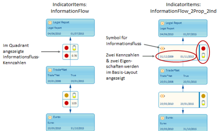
Abbildung: Für Verbindungselemente verfügbare Diagrammelementvorlagen
