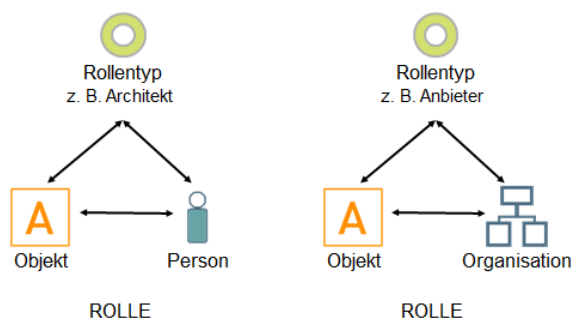
Abbildung: Beispiele für mögliche Definitionen einer Rolle
